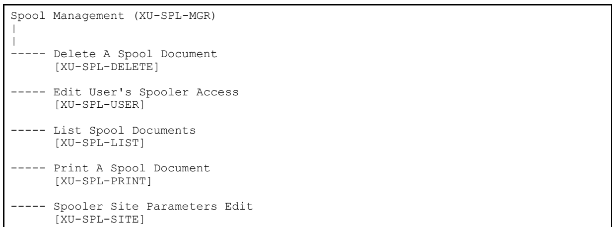
Figure 11. XU-SPL-MGR—Menu tree diagram
